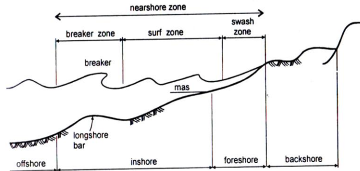
Gambar 1. Definisi dan batasan pantai
