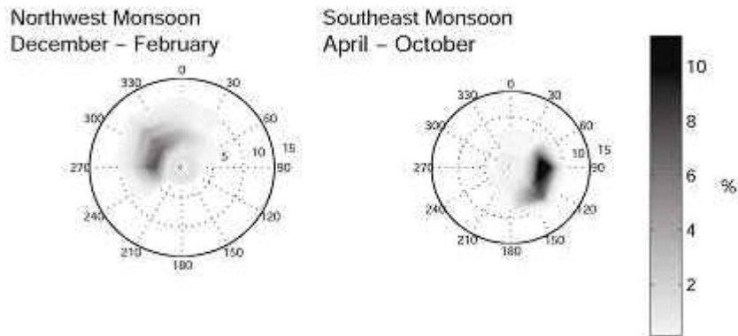
Gambar 4. Angin Dominan Berdasarkan musim di perairan Teluk Banten
