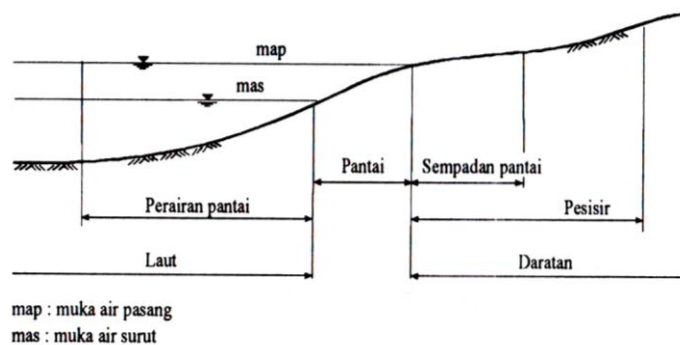
Gambar 2. Karakteristik gelombang di wilayah pantai
