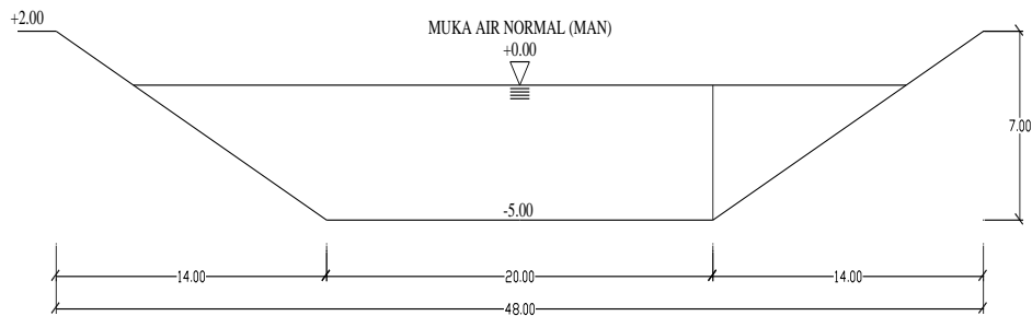
Gambar 8 Rencana Penampang Kanal
