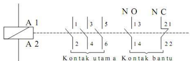
Gambar 15 Simbol kontak-kontak Kontaktor
