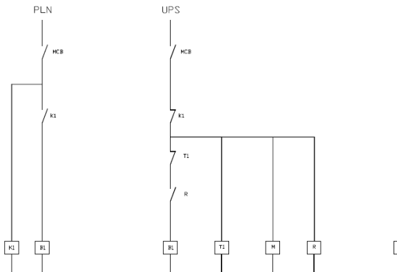
Gambar 8 Rangkaian control perangkat ATS
