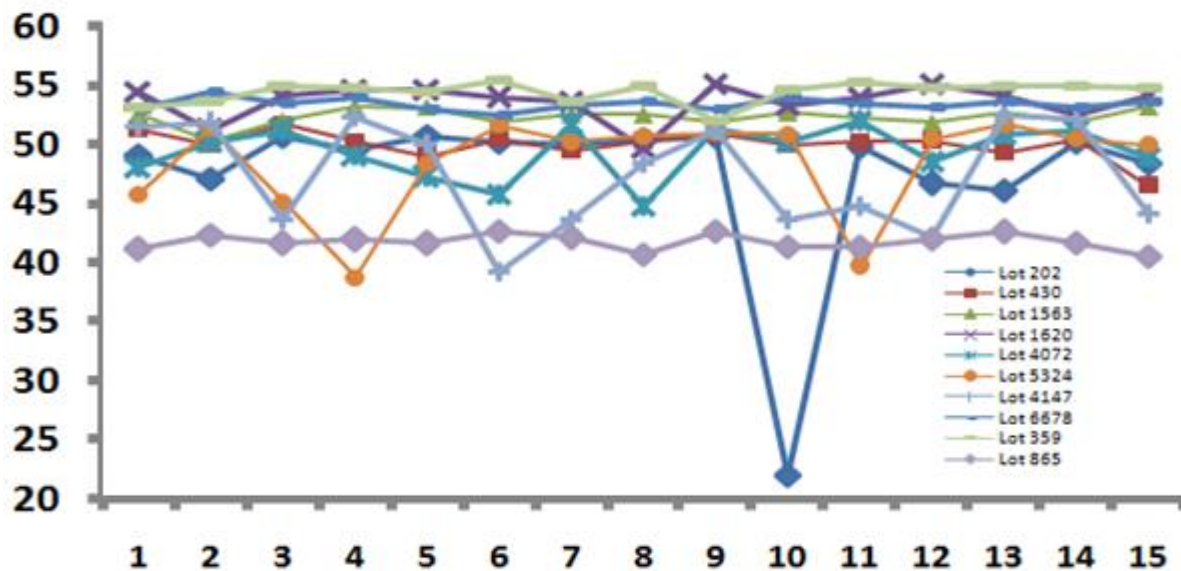
Gambar 1. Grafik variasi nilai kekerasan berdasarkan no plot produksi
