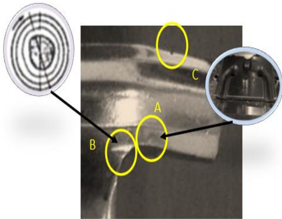
Gambar 5. Titik simulasi patahan bracket
