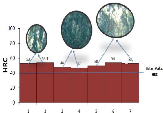
Gambar 6. Grafik nilai kekerasan terhadap matrik struktur mikro
