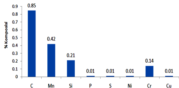
Gambar 3. Komposisi kimia baja karbon SK-5
