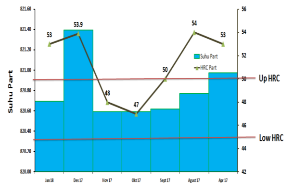
Gambar 7. Grafik nilai kekerasan terhadap perbedaan suhu produk pada proses austempering
