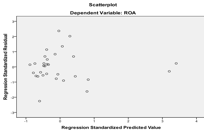
Gambar 4.3 Uji Heteroskedastisitas
